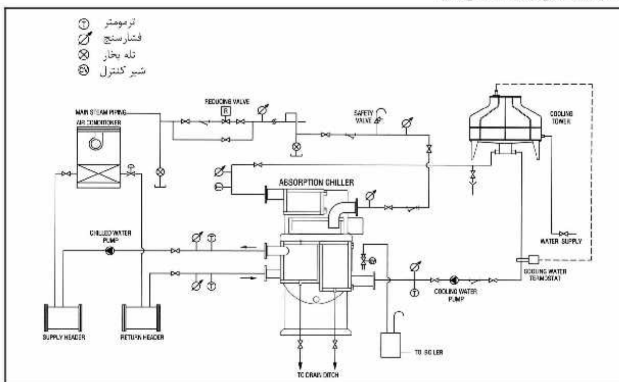
دیگرام لوله کشی چیلرهای جذبی بخار :
