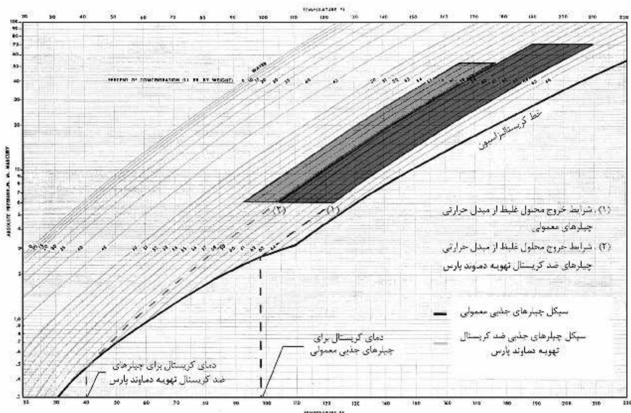
منحنی (Duhring diagram) چیلرهای جذبی آب گرم و بخار
