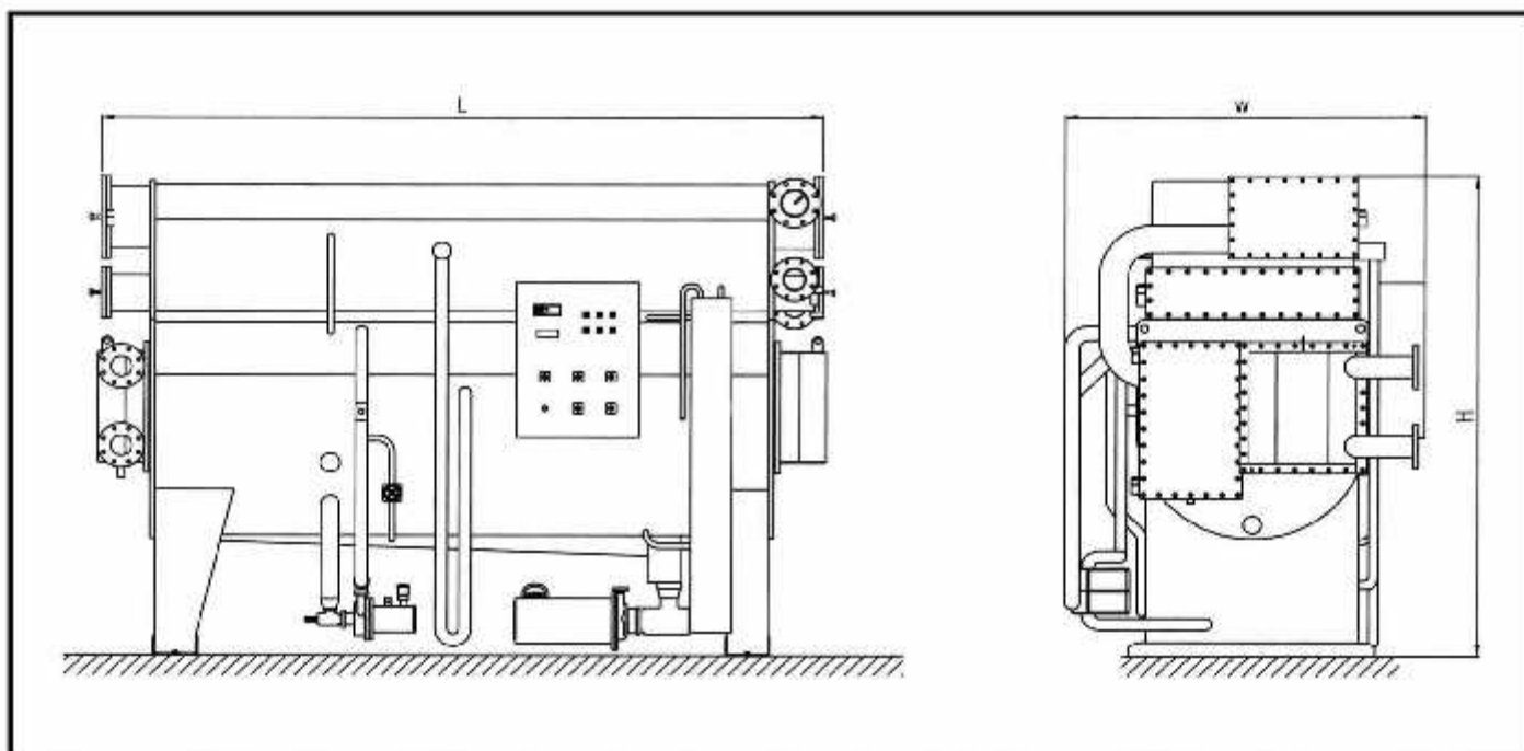
(جدول شماره ۲) ابعاد و اندازه های چیلر آب گرم ضد کربستال :
